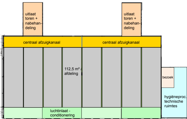
Grondplan van de nieuwe vleeskippenstal op het Proefbedrijf Plumveehouderij
