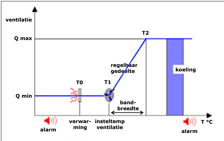
Schema klimaatregeling in functie van de staltemperatuur
