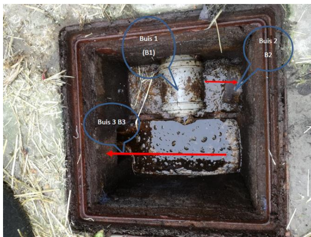
First-flushsysteem met B1 buis afkomstig van de mestvaalt, B2 overloop naar de mestkelder en B3 overloop naar de gracht.
